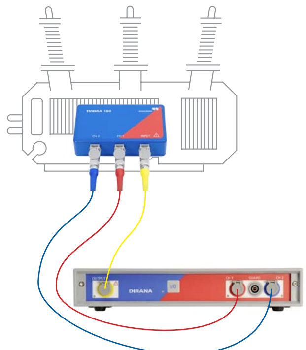
Das TMDRA 100 ist eine Demonstrationsbox zur Simulation dielektrischer Antwortkurven von Leistungstransformatoren
